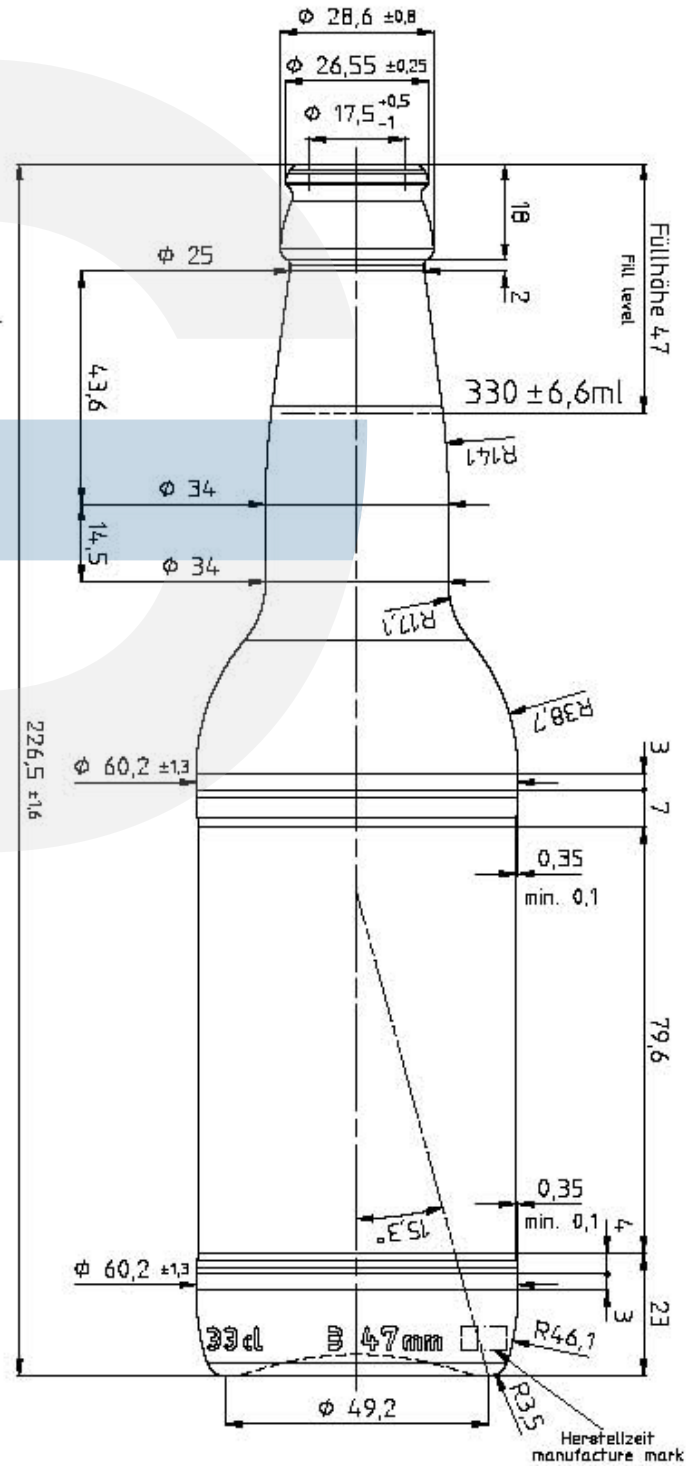
Standfläche geriffelt oder gekörnt bearing surface stippled or center punched
